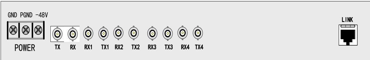
图 5-3 TF1004A -48V 电源后面板示意图
