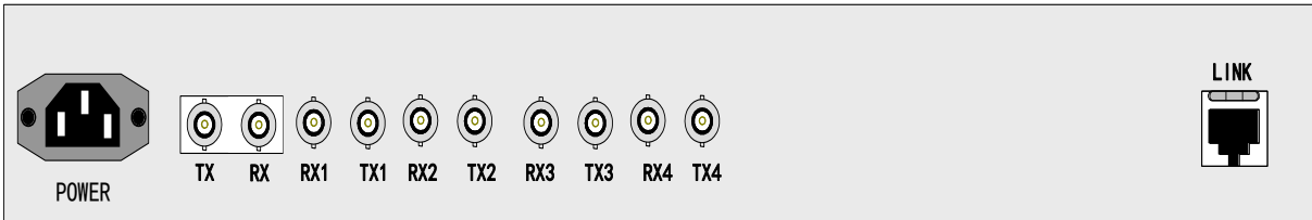
图 5-2 TF1004A 220V 电源后面板示意图
