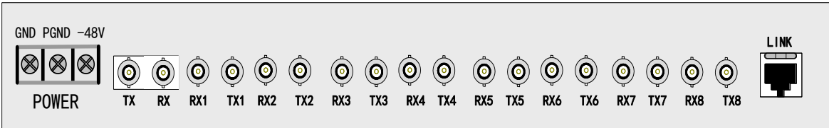
图 5-3 TF1004B -48V 电源后面板示意图
