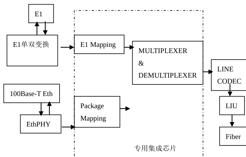
图 4-1 原理框图
