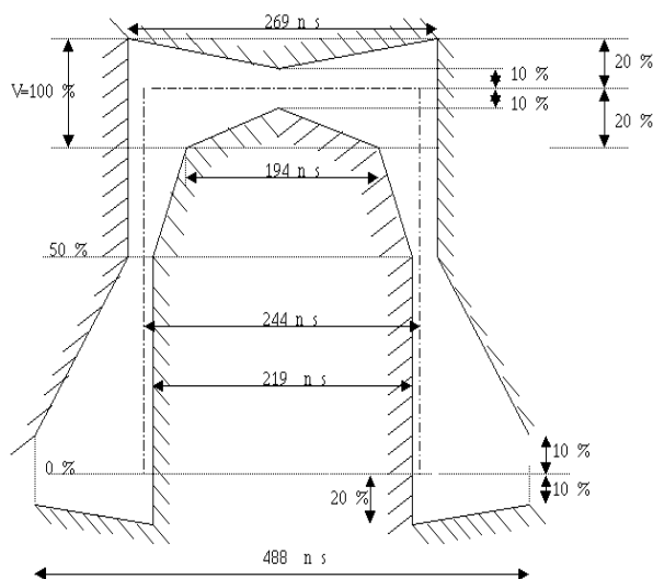
图 4-2 2M 线路码波形样板
