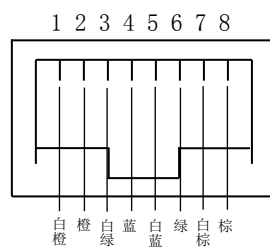
T568B
