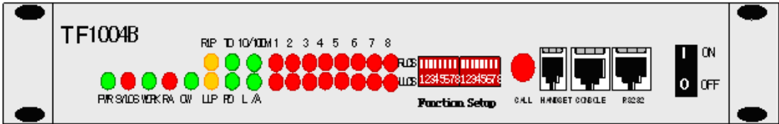
图 5-1 TF1004B 前面板示意图
