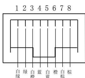
T568A
