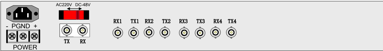
图 4 TF120C 后面板示意图
