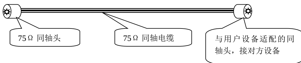
附图 2 75Ω 同轴接口连接的 E1 接口连线制做方法
