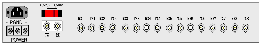
图 5 TF120D 后面板示意图
