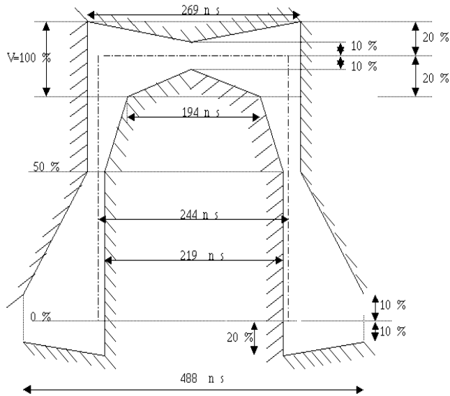
图 2 2M 线路码波型样板
