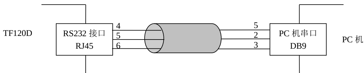
附图 1 RS232 接口连接线制作方法
