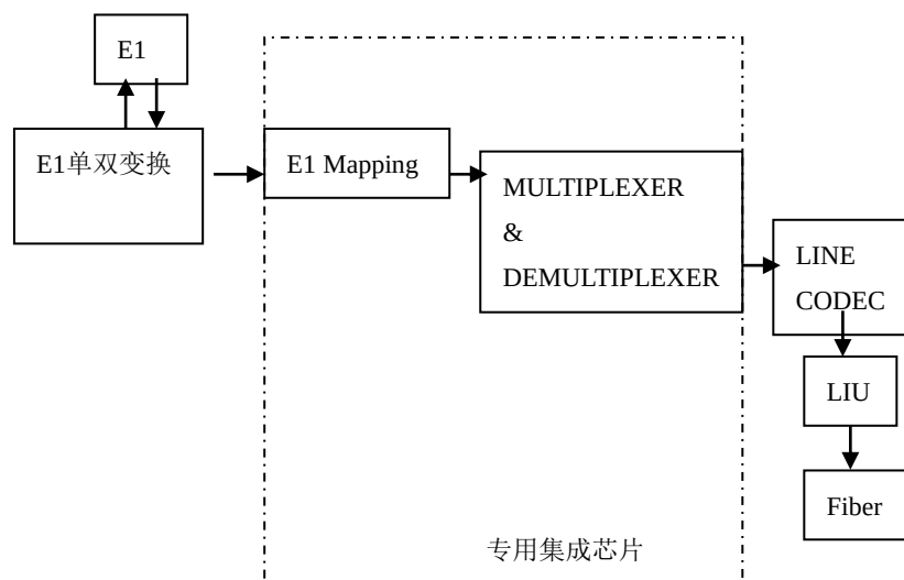
图 1 原理框图
