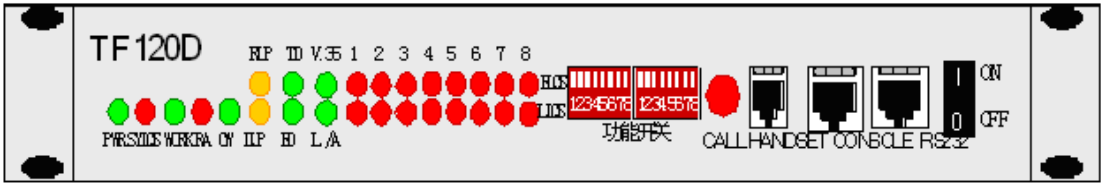
图 3 TF120D 光传输设备前面板
