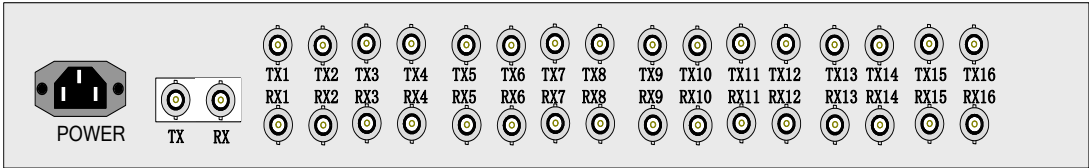
图 4 TF120H 220V 电源后面板示意图
