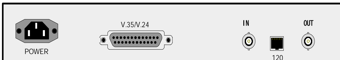
TF2000A E1/V. 35 转换设备后面板
