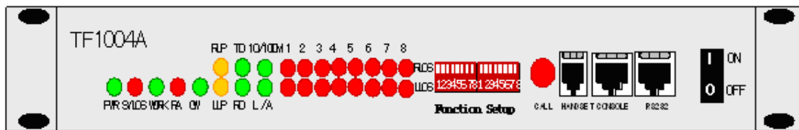
图 5-1 TF1004A 前面板示意图
