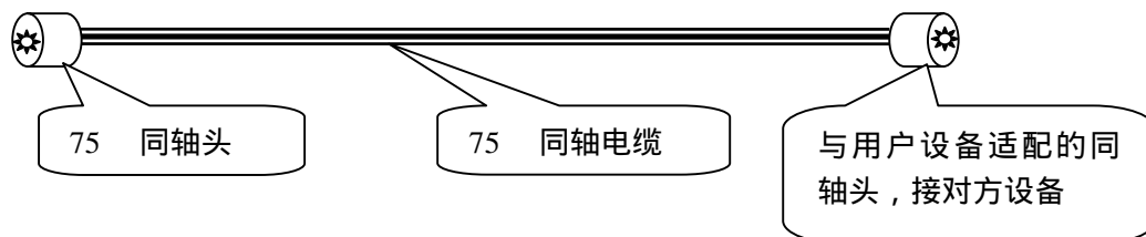
附图 1 75 同轴接口连接的 E1 接口连线制作方法
