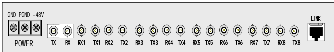
图 5-3 TF1004B -48V 电源后面板示意图
