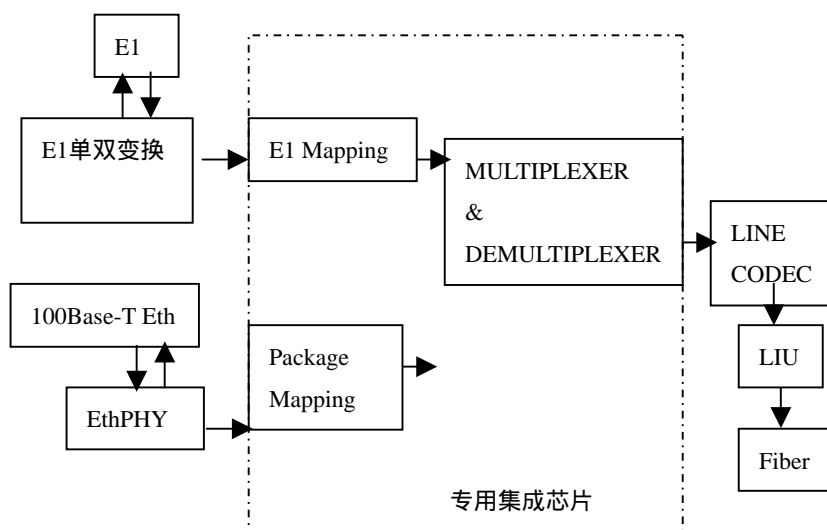
图 4-1 原理框图
