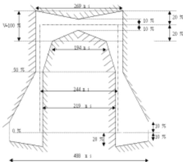
图 4-2 2M 线路码波型样板
