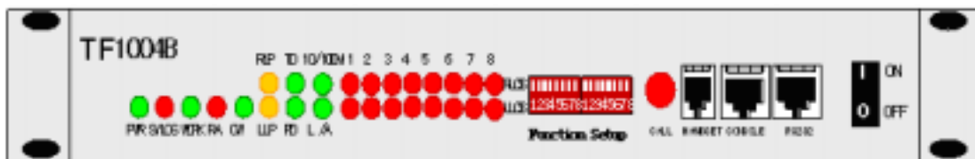
图 5-1 TF1004B 前面板示意图
