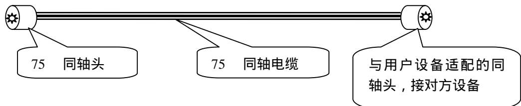
附图 2 75 同轴接口连接的 E1 接口连线制作方法
