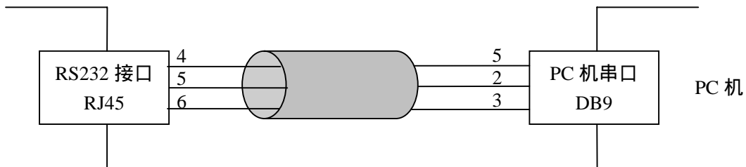
附图 1 RS232 接口连接线制作方法
