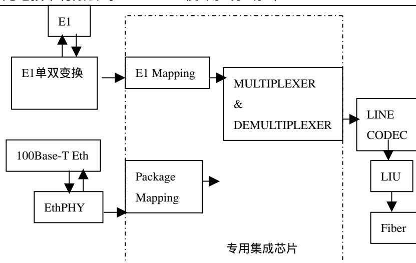
图 4-1 原理框图
