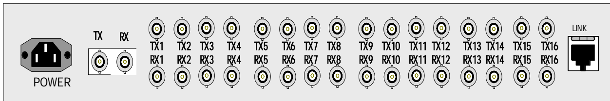
图 5-8 TF1004C 220V 电源后面板示意图
