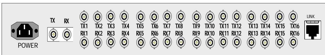
图 5-8 TF1004C 220V 电源后面板示意图
