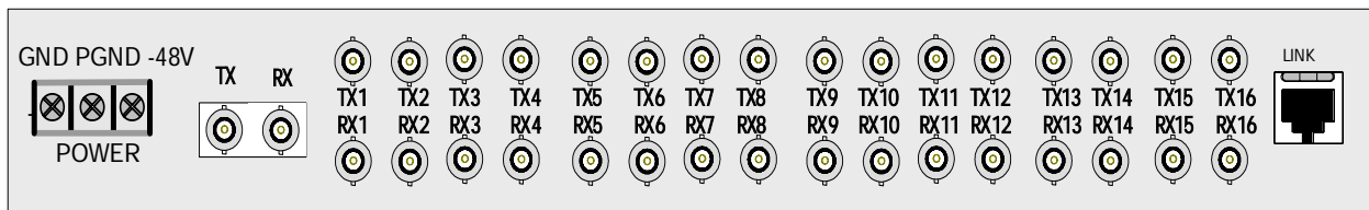
图 5-9 TF1004C -48V 电源后面板示意图
