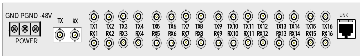
图 5-9 TF1004C -48V 电源后面板示意图
