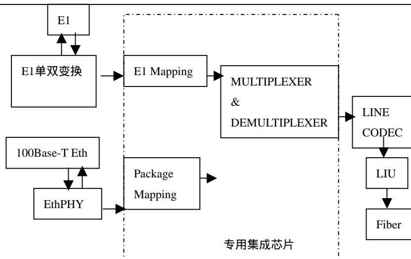
图 4-1 原理框图
