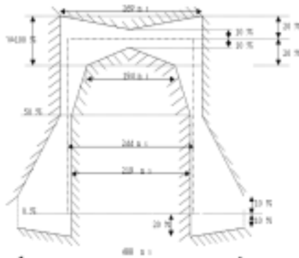
图 4-2 2M 线路码波形样板
