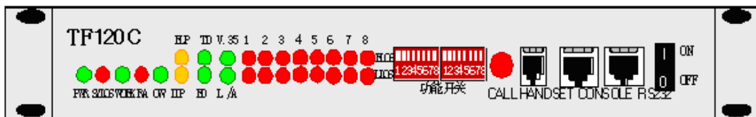
图 3 TF120C 光传输设备前面板
