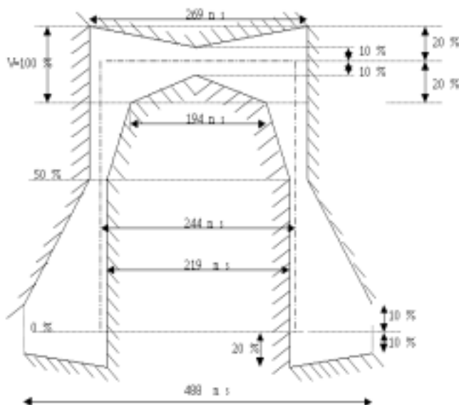
图 2 2M 线路码波形样板
