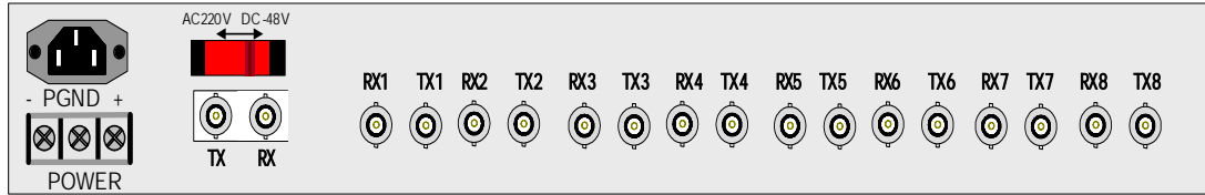
图 5 TF120D 后面板示意图
