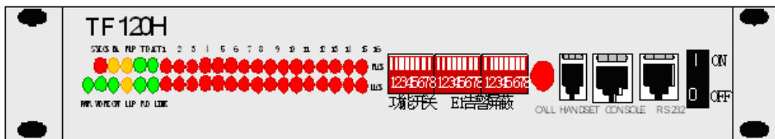
图 3 TF120H 光传输设备前面板
