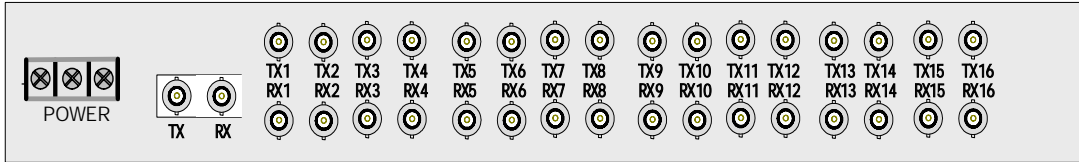
图 5 TF120H -48V 电源后面板示意图
