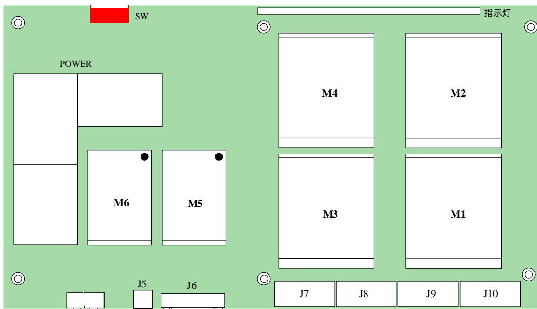
TF30TC 综合接入光端机主板平面图
