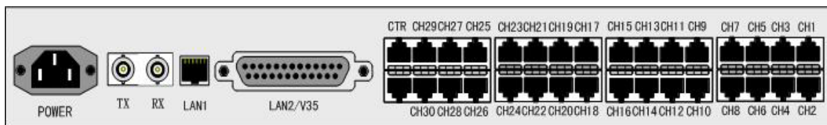
TF30TC 综合接入光端机后面板
