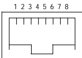
RJ45 插头
